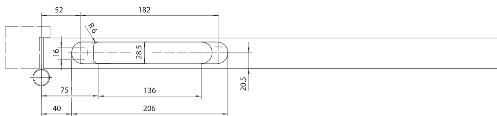
Obróbka skrzydła drzwiowego
