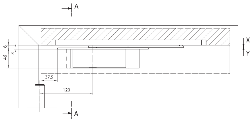
Przekrój wzdłużny
