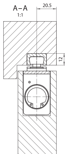
Przekrój poprzeczny
