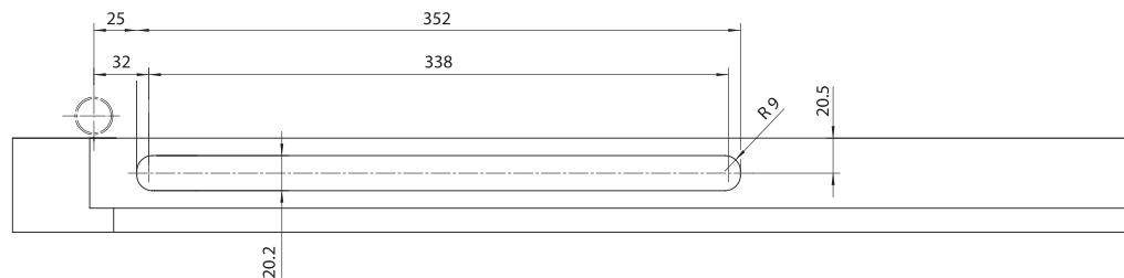
Obróbka ościeżnicy
